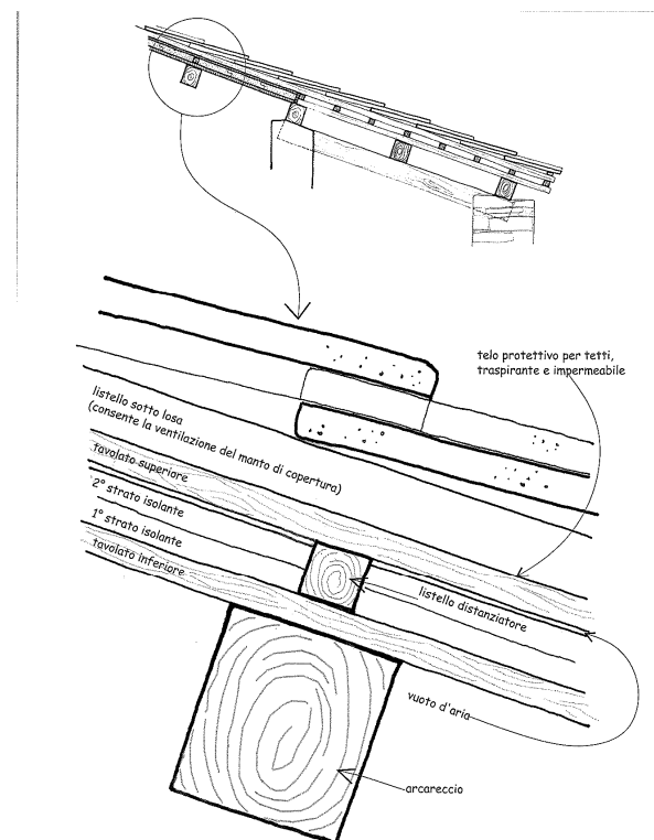
Copertura isolata e ventilata a falsi puntone.
